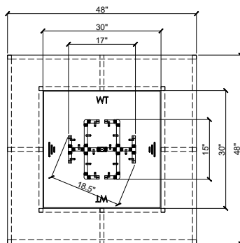
48" Top Elevation
