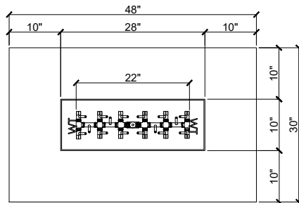
48" Top Elevation
