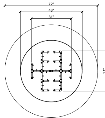
72" Top Elevation
