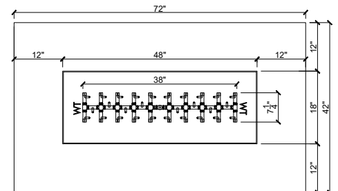
72" Top Elevation
