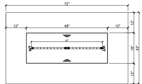
72" Top Elevation
