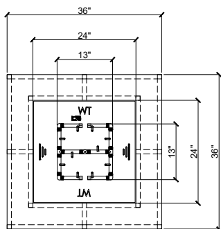
36" Top Elevation
